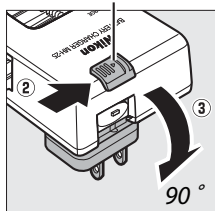
墙式适配器锁门
